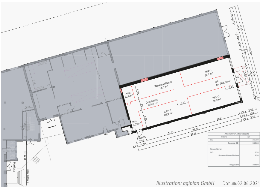
Abb. 15: Entwurfszeichnung eines Mikro-Depots
